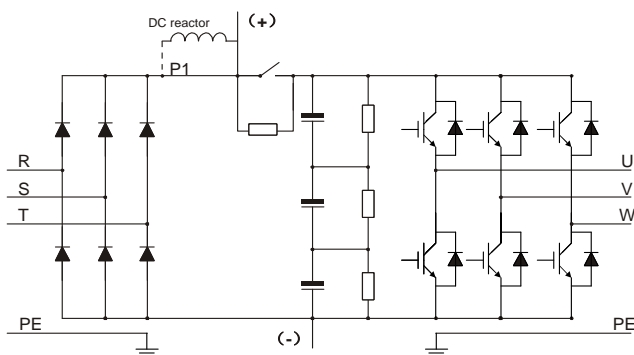
Рис 3.4 Схема силовой цепи 660В
